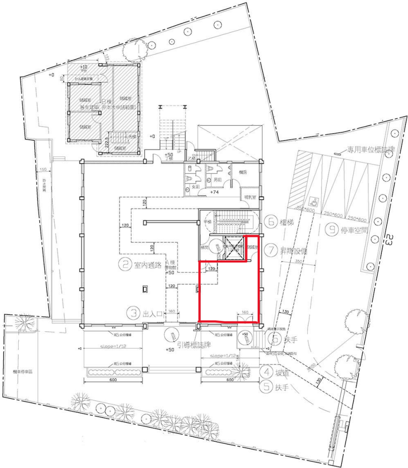
A棟一層平面圖 A1 S=1/100 A3 S=1/200
